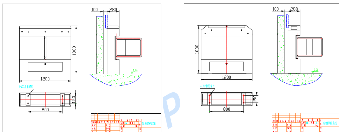
桥式圆角摆闸
