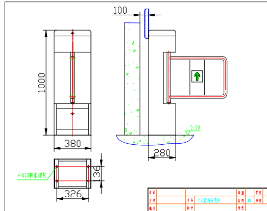
立式摆闸
