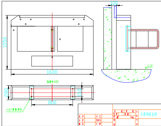
长摆闸
