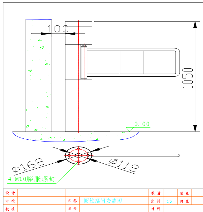
圆柱摆闸
